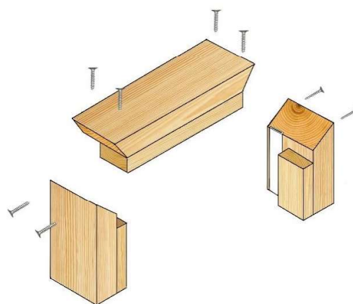
Mitre Joint
